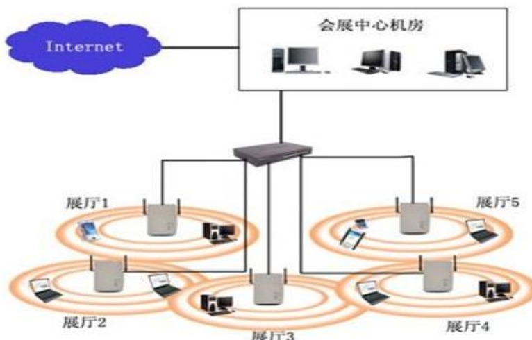
图3-2.会展中心应用架构
