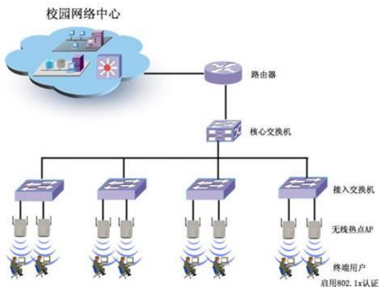
图3-1.校园应用架构
