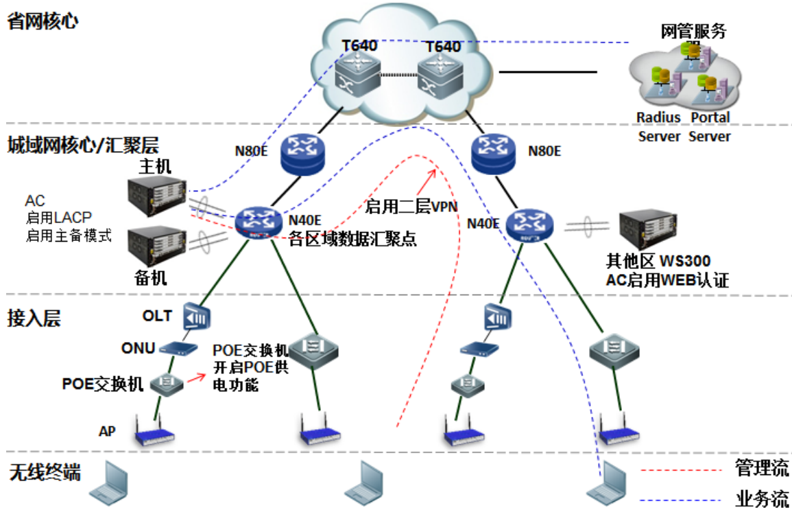
0 AP 模式网络某种架构
